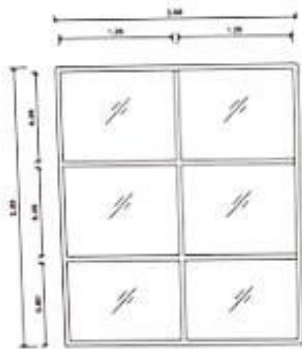
แบบขยาย 1
